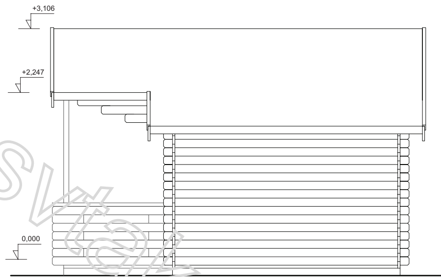
POHLED 4
