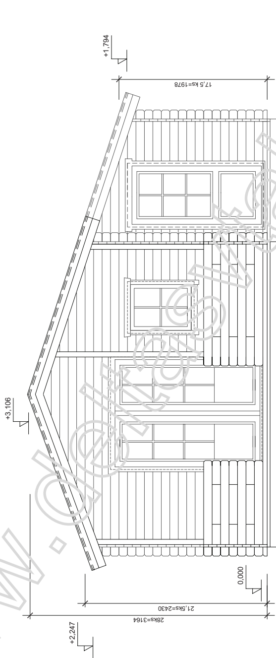
POHLED 1
